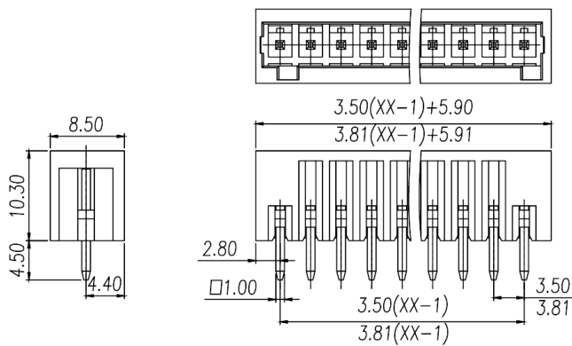
尺寸图 Dimensions
