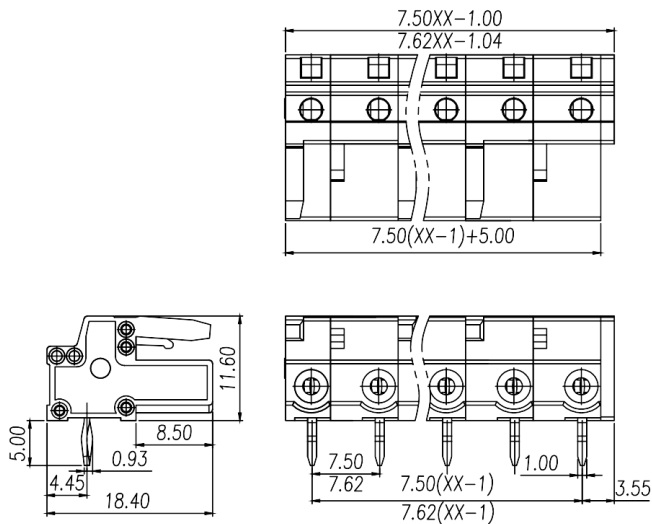
尺寸图 Dimensions
