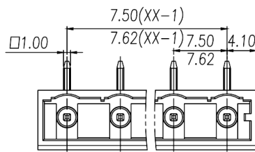
尺寸图 Dimensions
