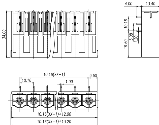
尺寸图 Dimensions
