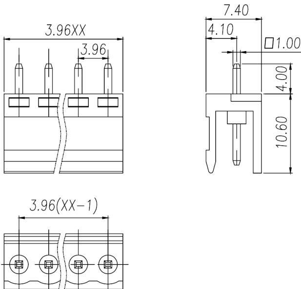
尺寸图 Dimensions
