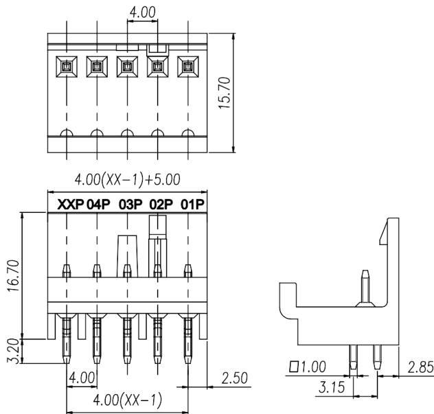
尺寸图 Dimensions
