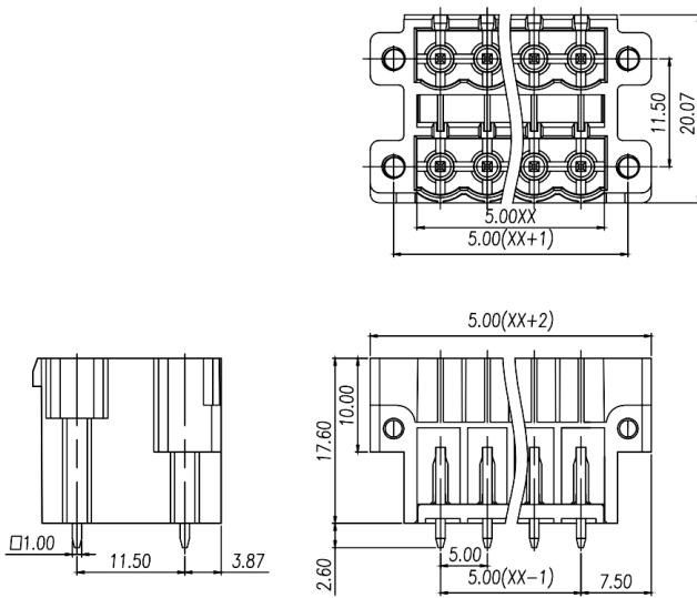
尺寸图 Dimensions
