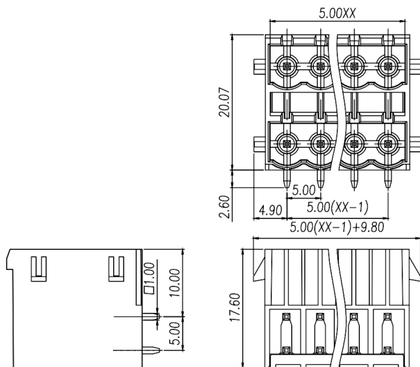
尺寸图 Dimensions
