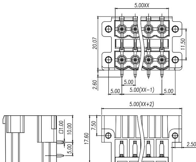
尺寸图 Dimensions
