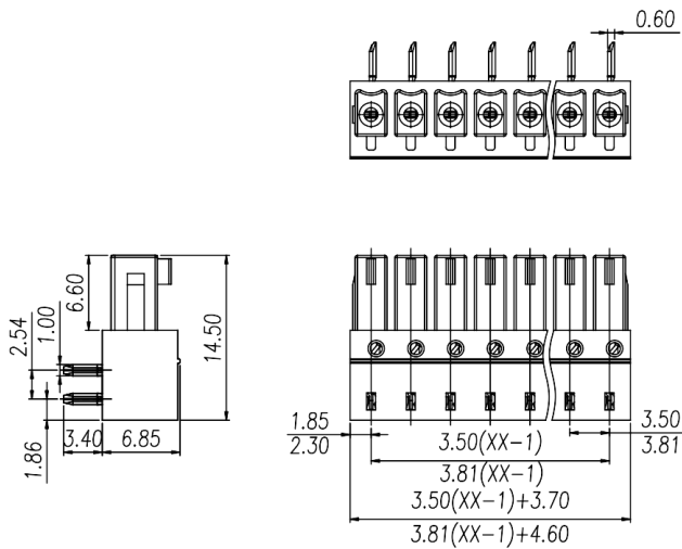
尺寸图 Dimensions
