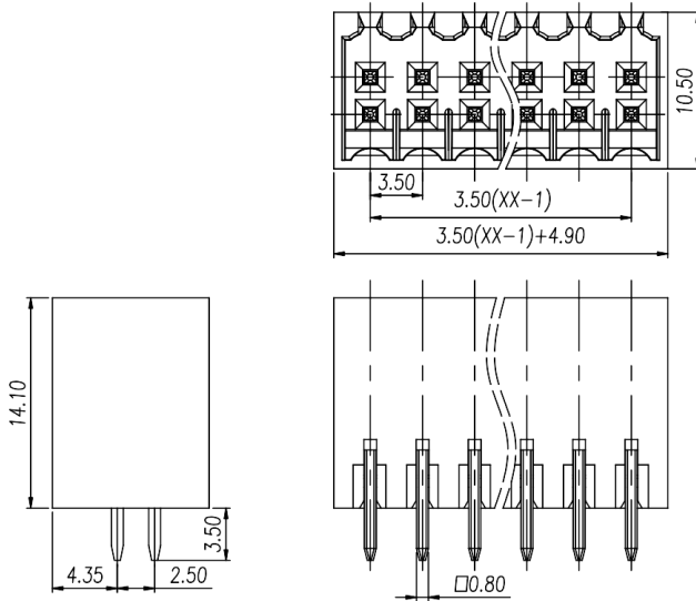
尺寸图 Dimensions
