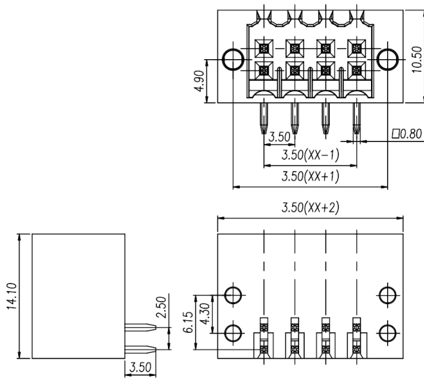
尺寸图 Dimensions
