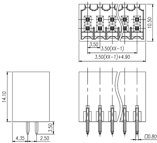
尺寸图 Dimensions
