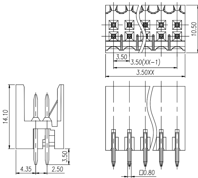
尺寸图 Dimensions
