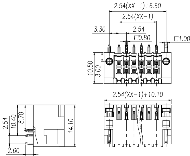
尺寸图 Dimensions
