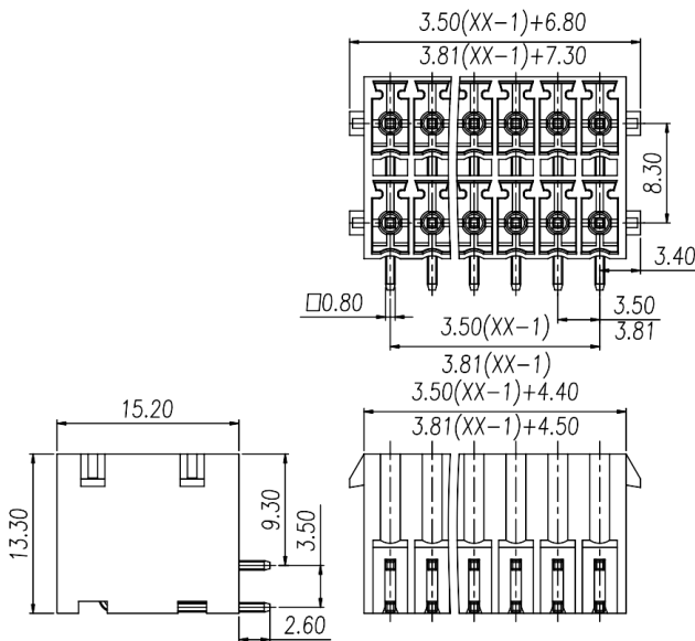
尺寸图 Dimensions
