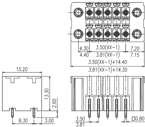
尺寸图 Dimensions
