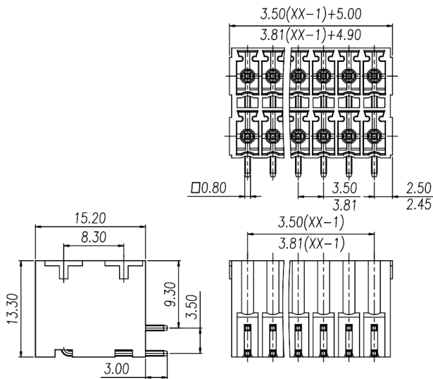
尺寸图 Dimensions
