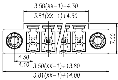
尺寸图 Dimensions
